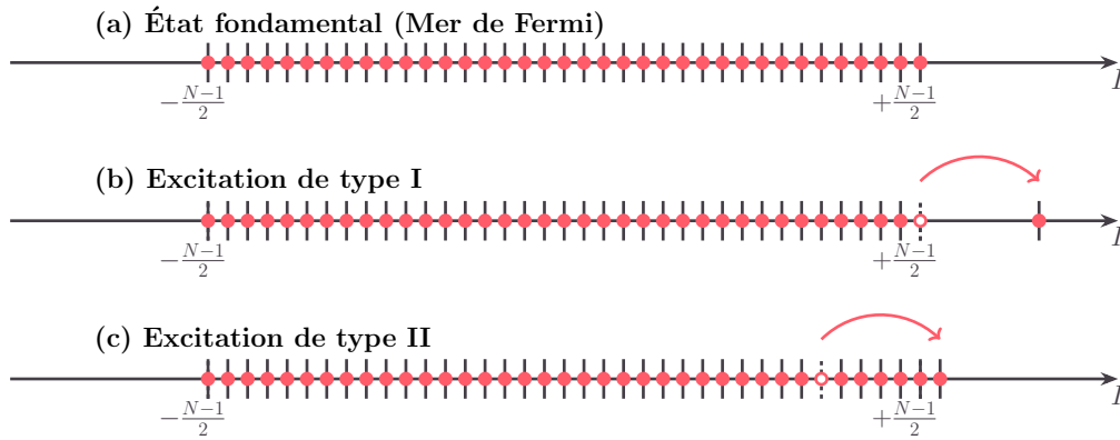
FIGURE I .2 – Représentation schématisée de la mer de Fermi pour un système de N particules : (a) distribution occupée à l'état fondamental, analogue à une mer de Fermi idéale ; (b) modification de cette distribution sous l'effet d'une excitation élémentaire de type I ; (c) modification correspondante en présence d'une excitation élémentaire de type II.
