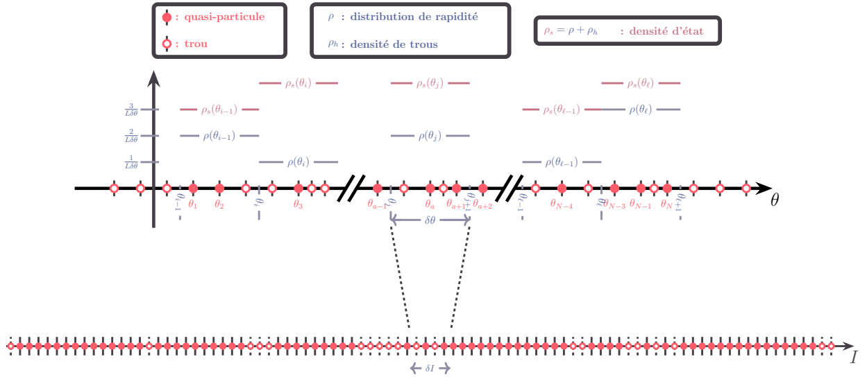
FIGURE I .3 – Illustration de la relation entre la densité d'états \rho_s(\theta) et les nombres quantiques fermioniques I_a . Les rapidités dans l'intervalle [\theta, \theta + \delta\theta] s'associent à un ensemble de nombres quantiques fermioniques situés dans [I, I + \delta I] . La densité d'états \rho_s se déduit alors de la relation \delta I \simeq L\rho_s(\theta)\delta\theta
